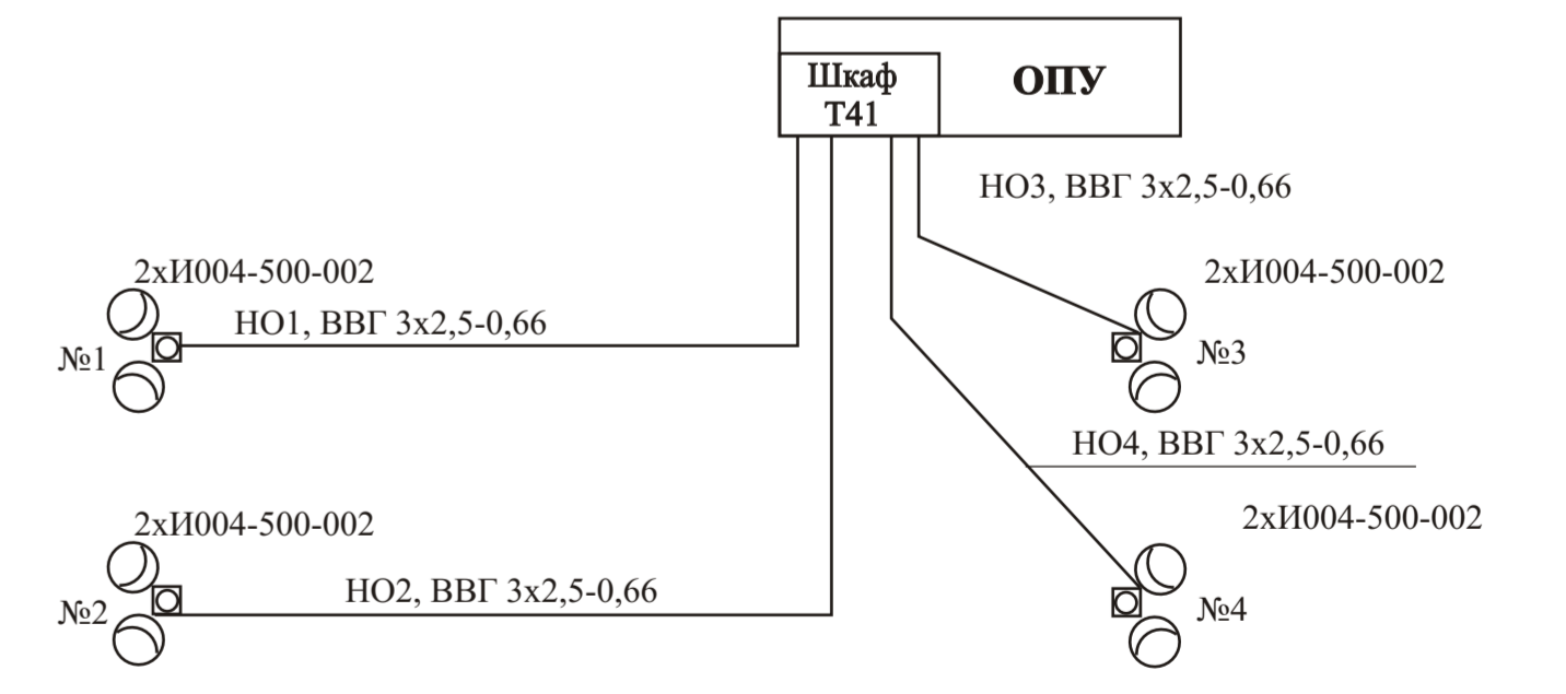
Схема управления наружным освещением
